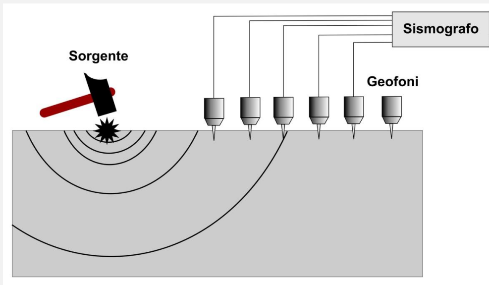
Figura 1. Stendimento sismico. Nel caso si utilizzi una sorgente ad impatto verticale (la classica martellata verticale) si acquisiranno dati utili all'analisi delle onde di Rayleigh (per fare questo si possono utilizzare geofoni verticali o geofoni orizzontali con asse allineato con lo stendimento – vedi oltre). Nel caso si utilizzino invece geofoni a componente orizzontale con asse perpendicolare allo stendimento e sorgente di taglio si otterrà un dataset utile all'analisi delle onde di Love e della rifrazione SH (vedi Figura 2).
